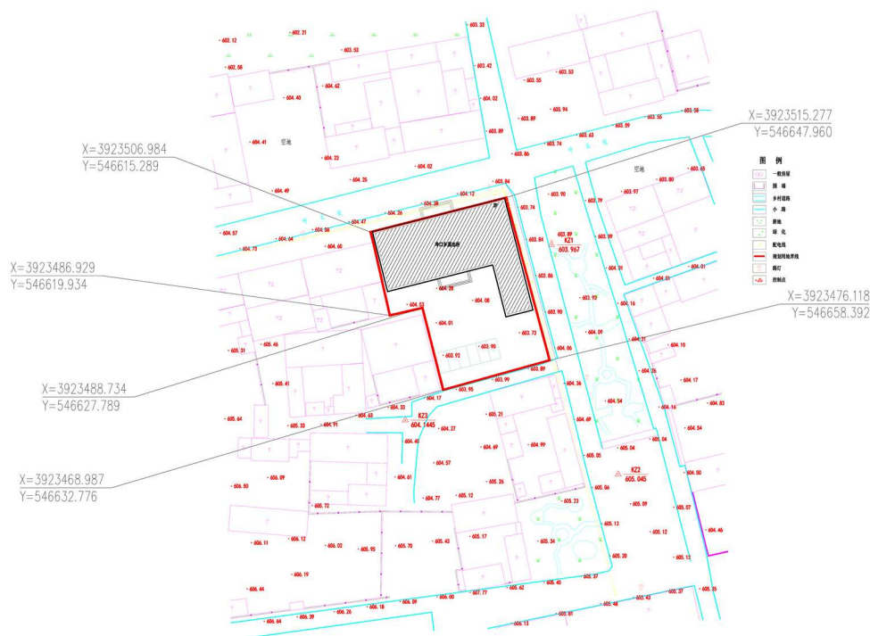
绛县冷口乡派出所建设项目用地与规划选址布置图
